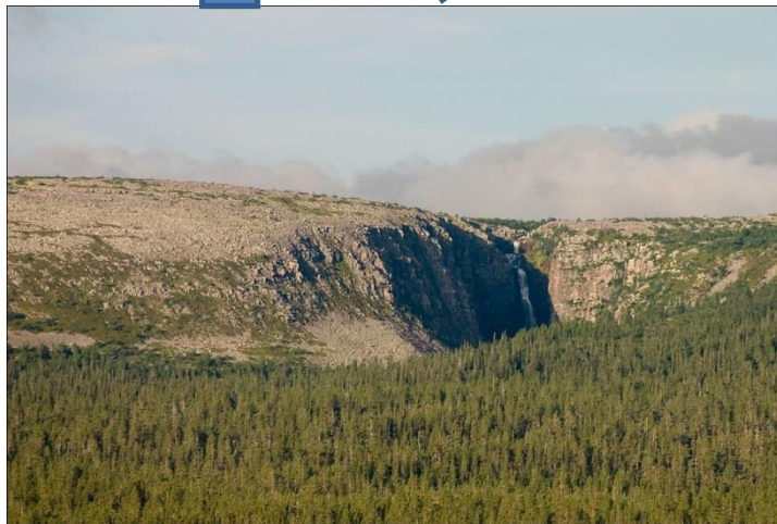
A. MS_Fulufjället_empirical
